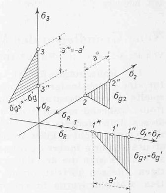
Bild 2. Axonometrische Darstellung der Teilchen 1'', 2'', 3'' in den Seitenflächen des Einheitswürfels und der Gitterspannungen \sigma_{g1}, \sigma_{g2}, \sigma_{g3} nach einem einseitigen Fließen in Richtung 1 an der zweiten Fließgrenze \sigma_1 = \sigma_f entsprechend \sigma_{g1} = \sigma_{g'} , \sigma_{g3} = -\sigma_{g'}
